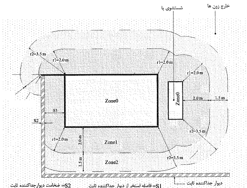
شکل ۱۳-۱۰-۳: طرحواره ابعاد مناطق (zone) استخر، با دیوار جداکننده ثابت حداقل به ارتفاع ۲/۵ متر (دید از بالا)
