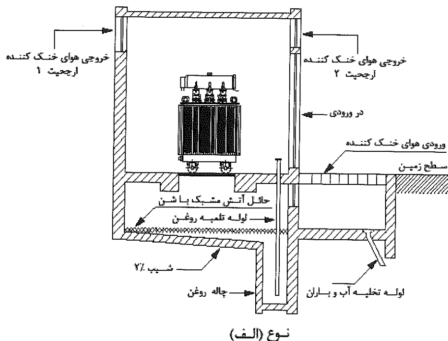
شکل ۵-۱۳-۳-۲: نوع الف) - طرحواره مقطع قائم اتاق ترانسفورماتور روغنی با تهویه مکانیکی و هم سطح زمین
