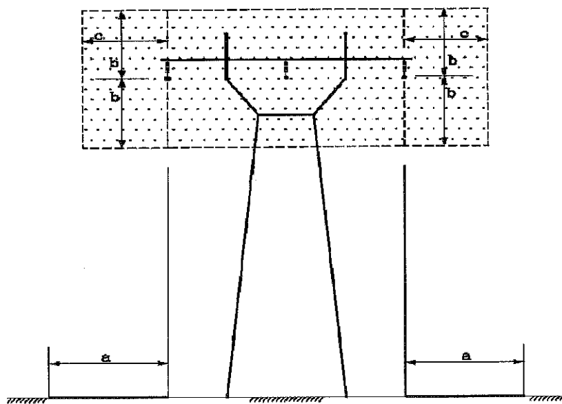
شکل پ ۲-۱-۲ خط هوایی فشار قوی (۶۳ کیلوولت و بالاتر)
